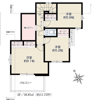
間取図
