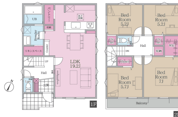
1号棟間取図
