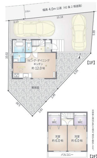
間取図
