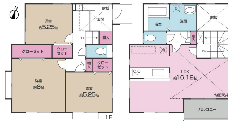
間取図
