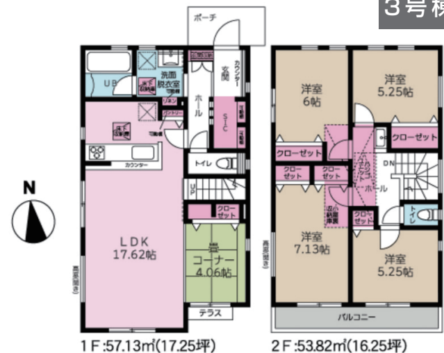
3号棟間取図
