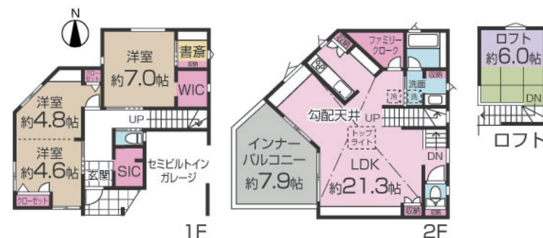
間取図
